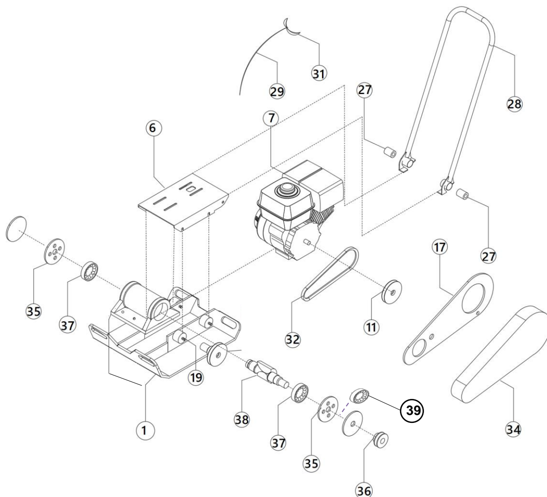
Despiece referencial de PC5050F
